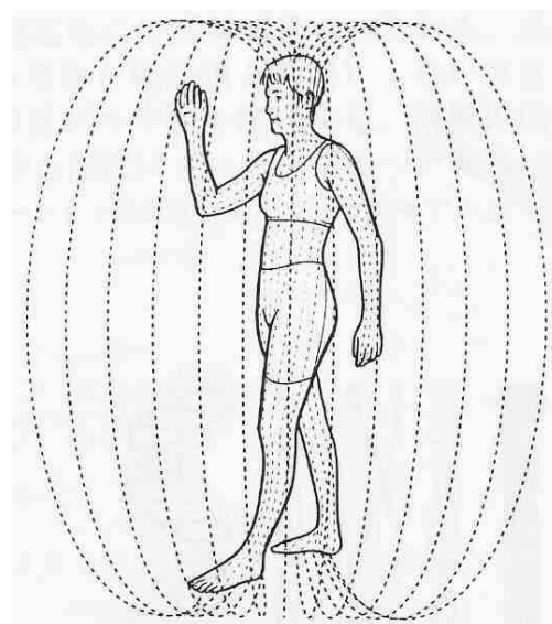
図 2 人体全体からの磁場形態
